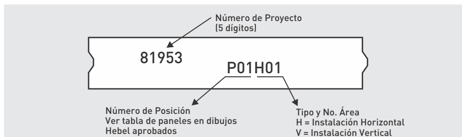
Fig. 5: Identificación de Panel Hebel para muro.
